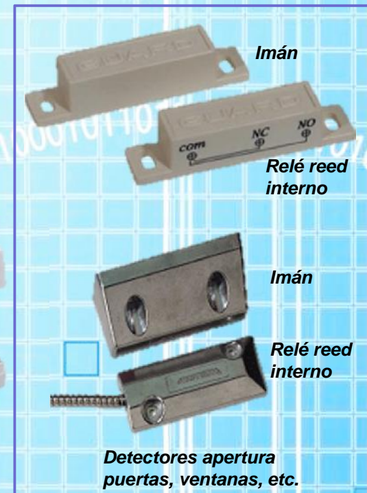
Relé 'reed'
