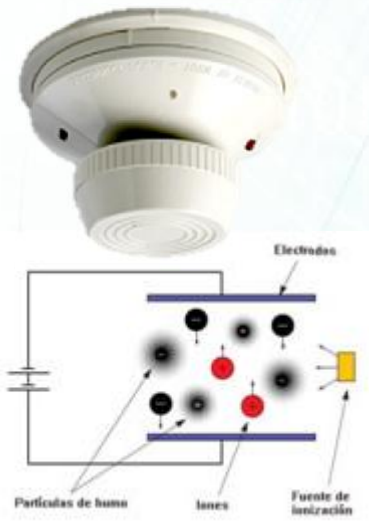
Detector iónico de humo
