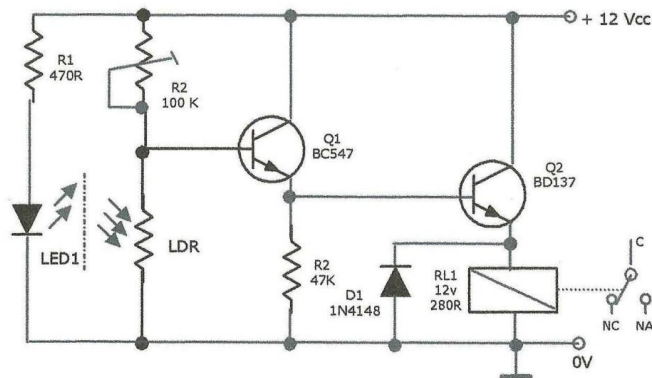
INTERRUPTOR POR OBSTRUCCIÓN
