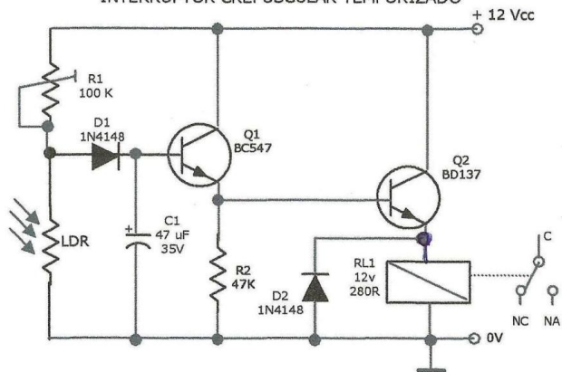
INTERRUPTOR CREPUSCULAR TEMPORIZADO
